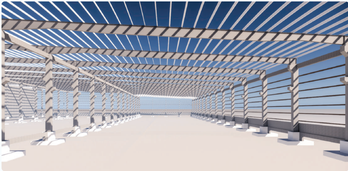
拼接混凝土柱、钢结构系统3D设计模型
