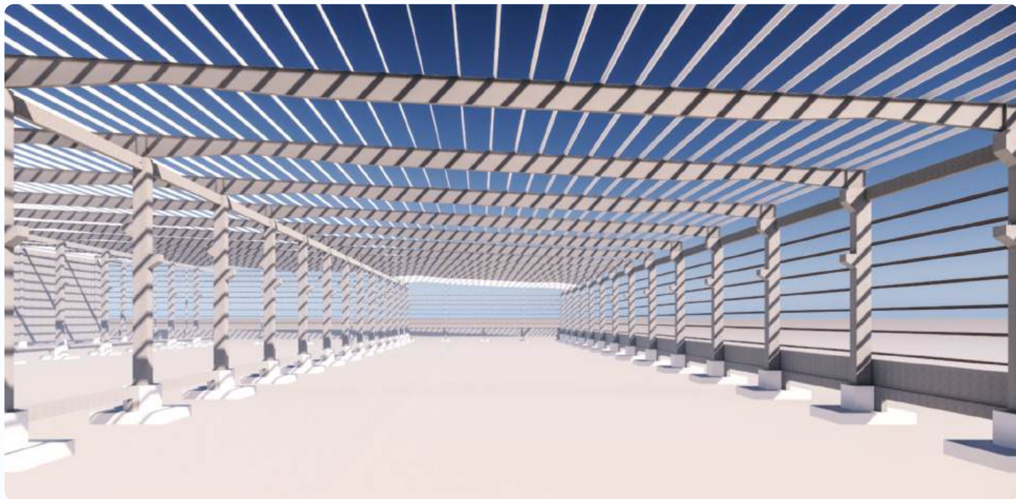
Mô hình 3D thiết kế cột bê tông lắp ghép, hệ kết cấu thép
